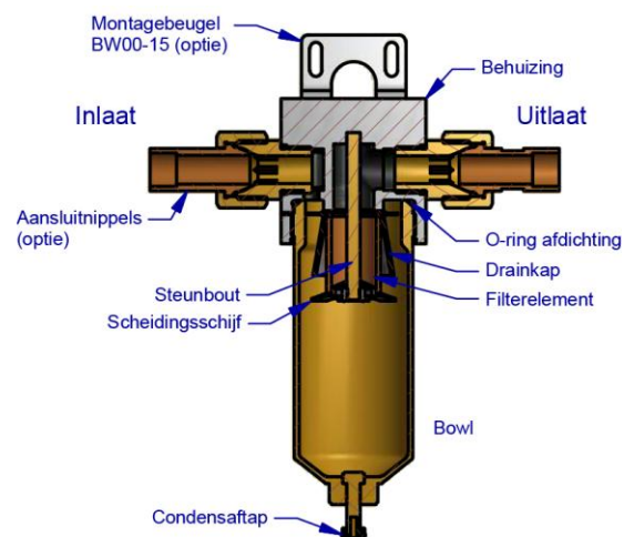
Doorsnede F445-03/4E/GL15
